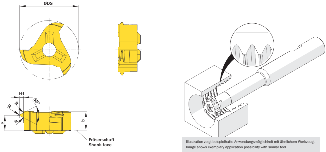
Abbildung zeigt / Drawing shows: U18.BS14.02 M
