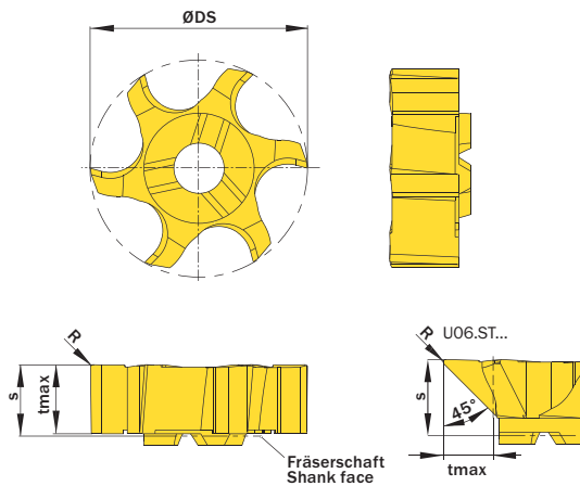
Abbildung zeigt / Drawing shows: U06.PL55.020.18 Y
