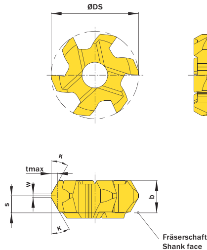
Abbildung zeigt / Drawing shows: P06.3030.02.10 F
